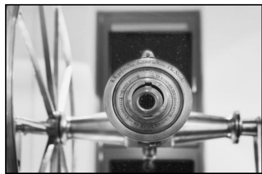
Το μεσημβρινό τηλεσκόπιο Starke. Χρησιμοποιήθηκε για τη μέτρηση του χρόνου από το Αστεροσκοπείο από το 1846 έως το 1900. (Φωτο: Κων/νος Γεωργιάδης)
